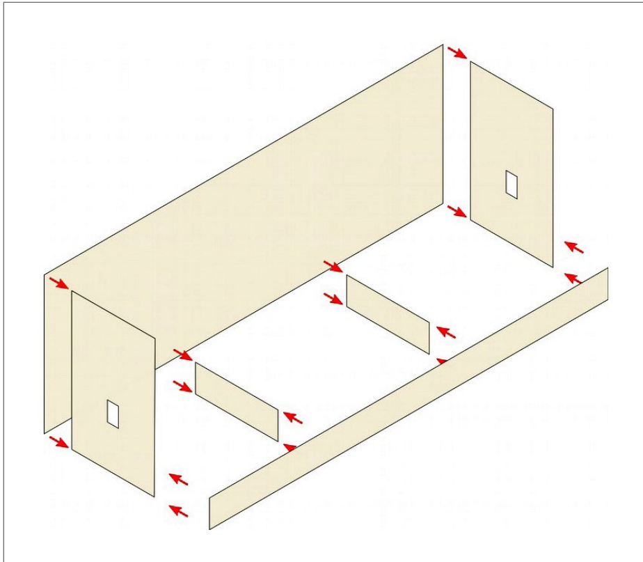
9. Module frame.
